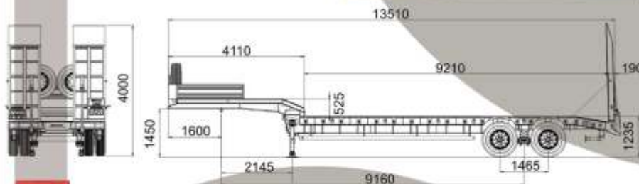
Rampas traseiras (2) movidas através de cilindros hidráulicos, com deslocamento lateral hidráulico e comandadas por distribuidor hidráulico de alavancas
