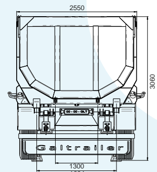
Pare-chocs à l'arrière rabattable
